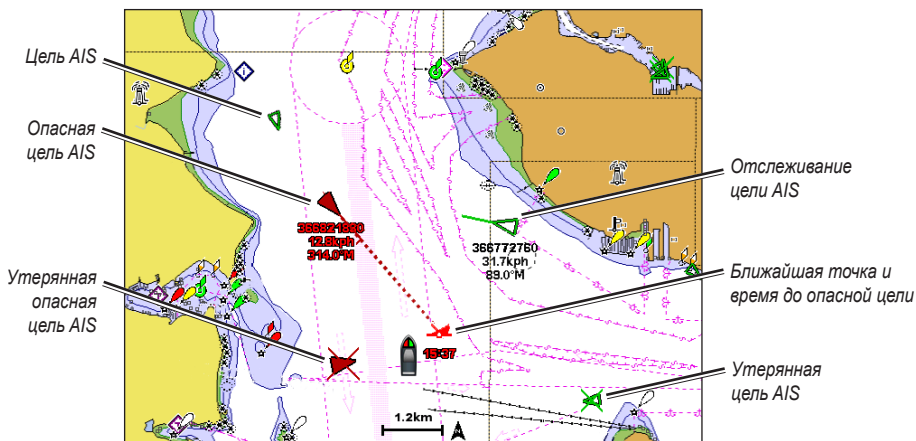
Навешение AIS на навигационной карте
